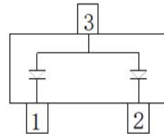
BAS70-06HQ
